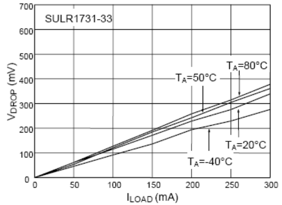
Fig. 2 V_{DROP} vs. I_{LOAD}
