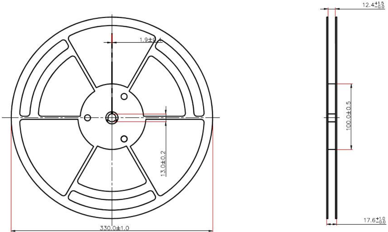
Fig 4. Reel dimensions
